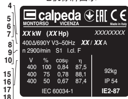
电机标牌图示
